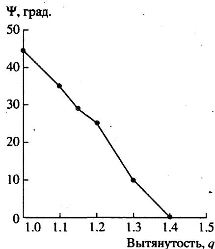
Рис. 5. Зависимость угла ориентации “легкой оси” \Psi относительно удлиненного ребра зерна от его вытянутости q .
