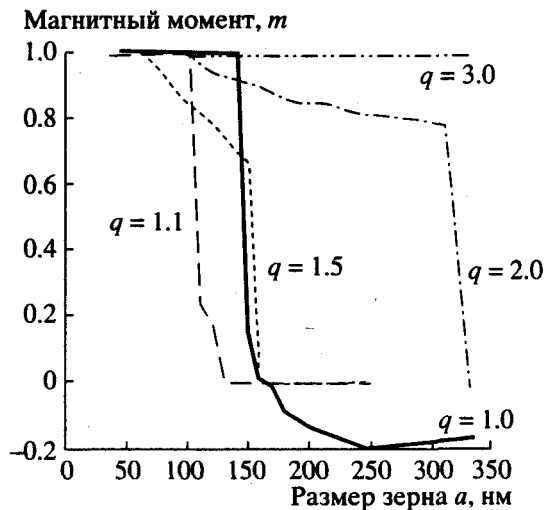
Рис. 3. Зависимость магнитного момента зерна от размера a и вытянутости q .
