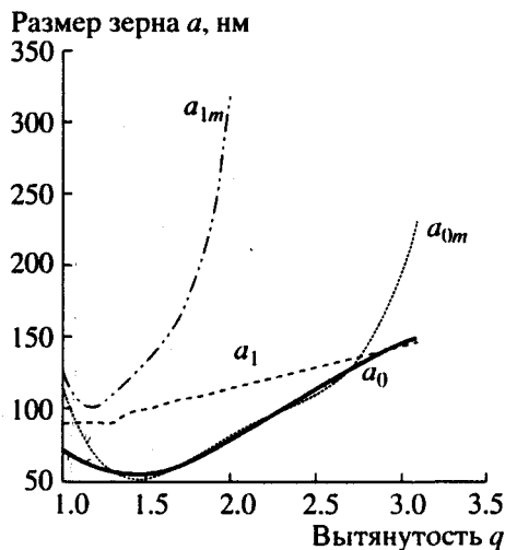
Рис. 4. Зависимость размера однодоменности a_0 , максимального размера с однородным распределением намагниченности a_{0m} , размера квазиоднодоменного a_1 и максимального размера квазиоднодоменного состояния a_{1m} от вытянутости зерна q .
