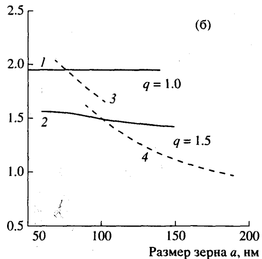
Рис. 2. Зависимость энергии зерна \varepsilon от его размера a и вытянутости q при различных исходных состояниях: а – с однородным распределением магнитного момента; б – с однородным (кривые 1, 2) и с неоднородным распределением магнитного момента (кривые 3, 4).
