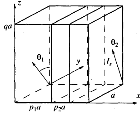
Рис. 1. Иллюстрация описываемой модели.
